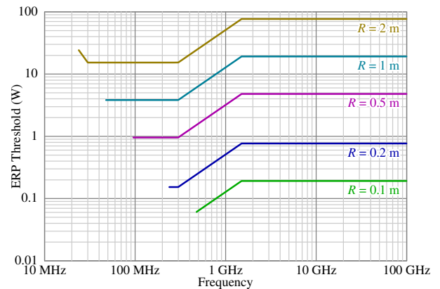
図 15: ERP の閾値のカーブの例 (47 CFR 1.1307 (b)(3)(i)(C) Table 1 (表 5) に基づく)
