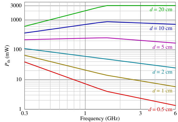
図 16: P_{\text{th}} のカーブの例 (§8.1.1.2 で示した式に基づく)
