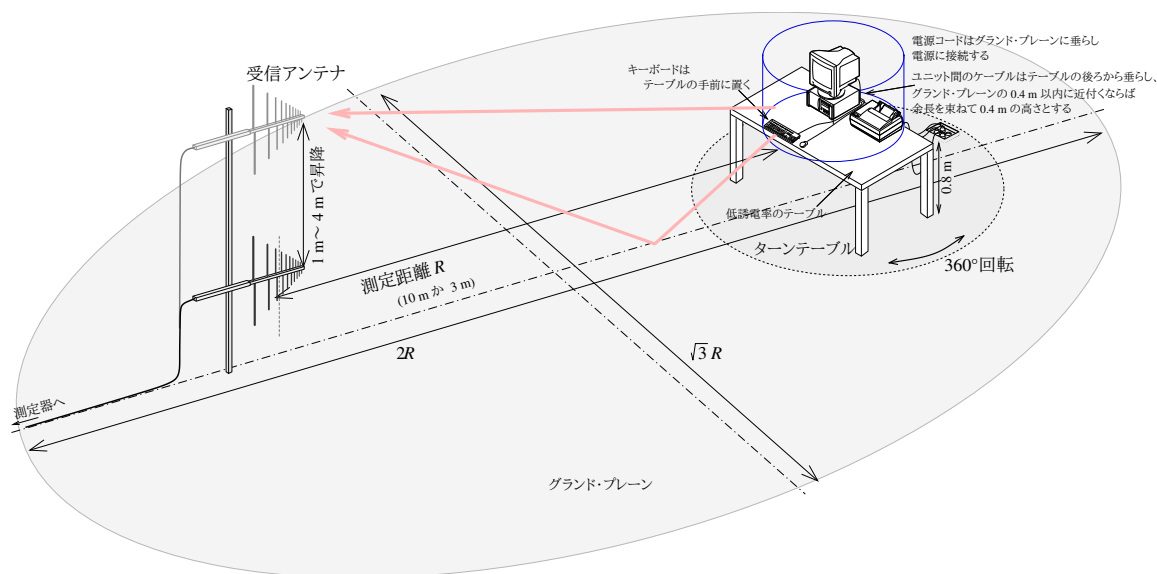
図 6: OATS での放射エミッション測定の設定アップのイメージ (30~1000 MHz)
